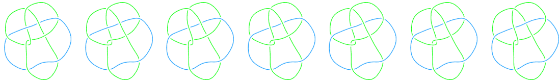
L10n44
