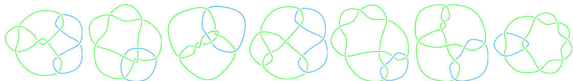
L9a8
