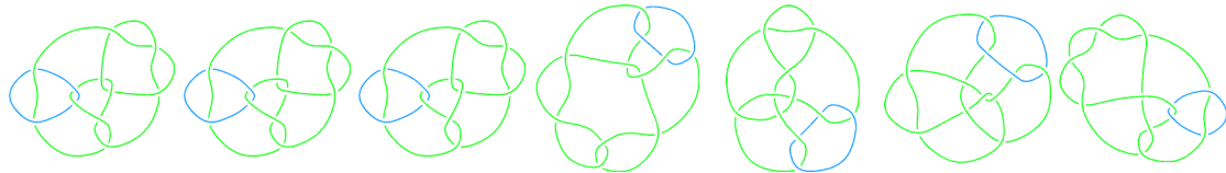
L11n62
