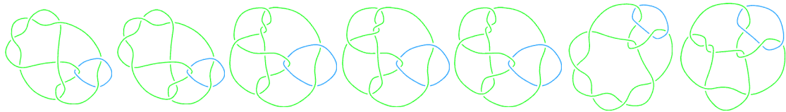
L11n69
