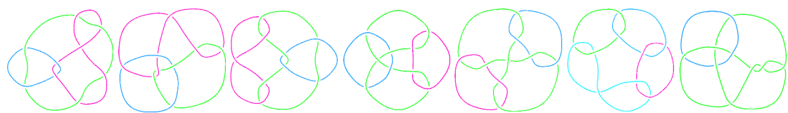
L9a50
