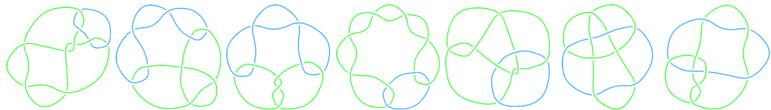
L9a15
