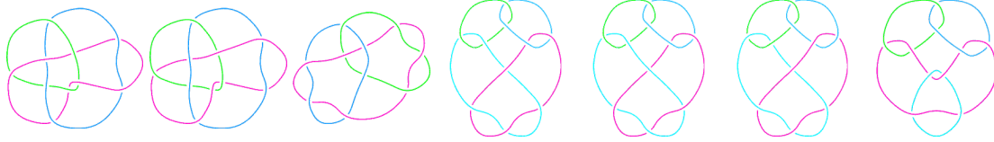
L10n93
