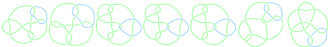
L10n23 L10n24 L10n25 L10n26 L10n27 L10n28 L10n29
