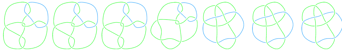
L9n9
