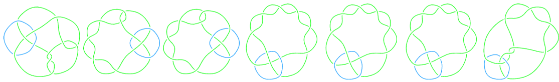
L11n41
