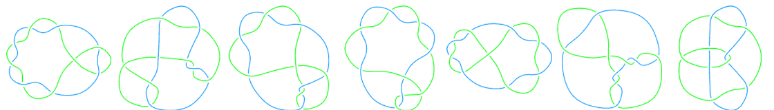
L9a36
