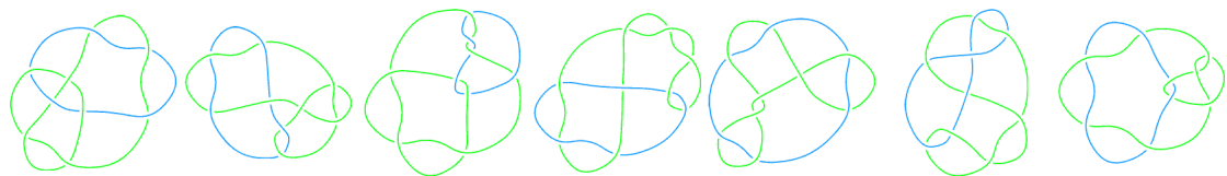
L9a22
