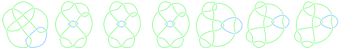
L11n90
