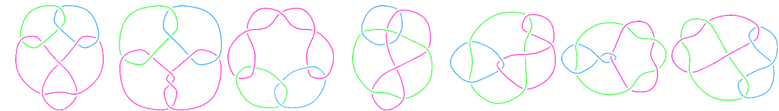
L9a43
