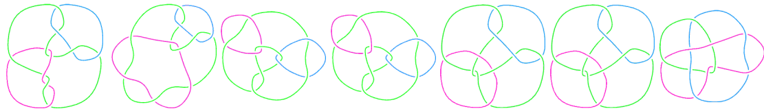
L10n86
