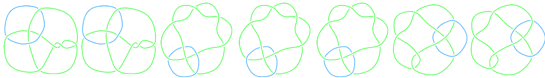
L9n2
