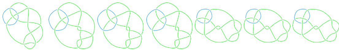
L11n6
