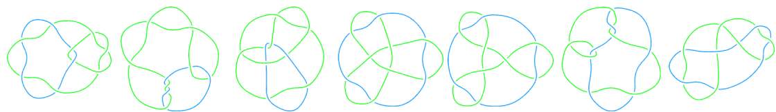
L9a29
