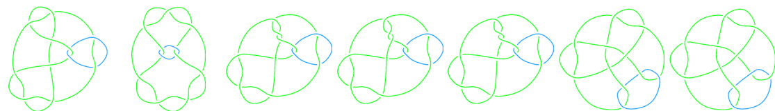
L11n97
